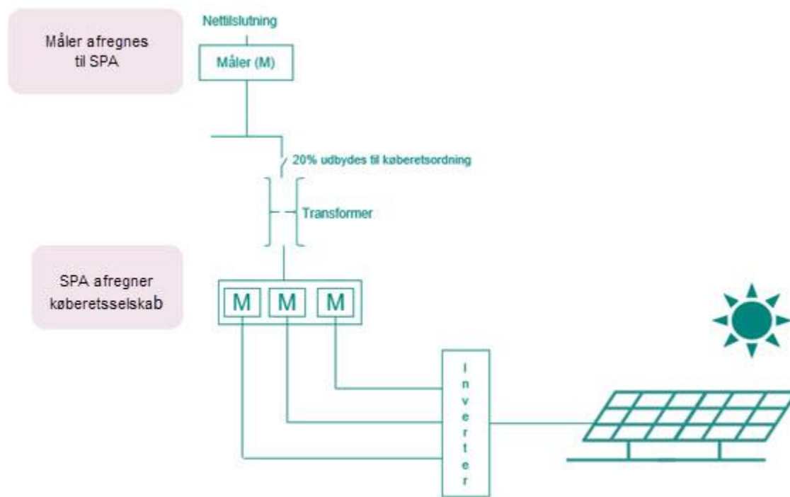
Figur 2 Skematisk illustration af måling af el fra Køberetsselskabet (SPRF = Solar Park Agersted Aps)
